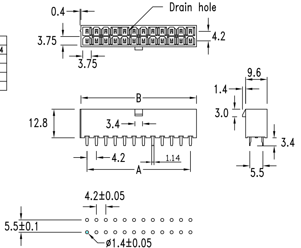
P.C.B. hole dimensions
